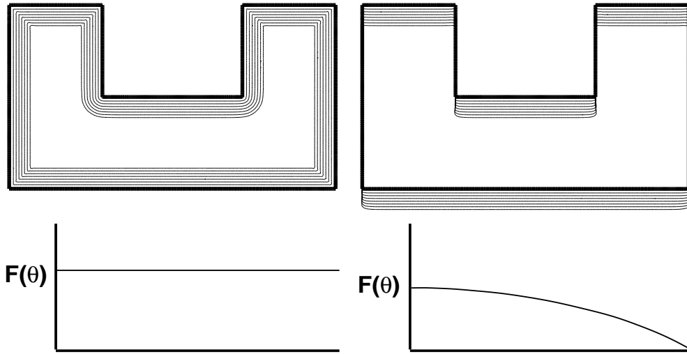
Fig. 24a. F(\theta) = 1 .
