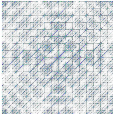
(d) 10 iterations
